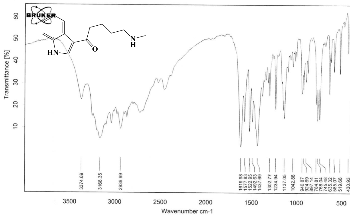
FT-IR SPECTRUM
