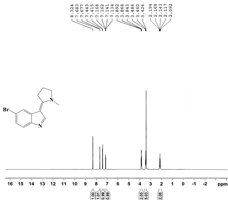
^1\text{H} -NMR SPECTRUM
