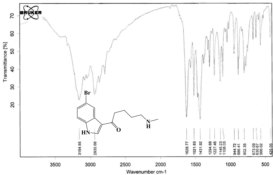
FT-IR SPECTRUM
