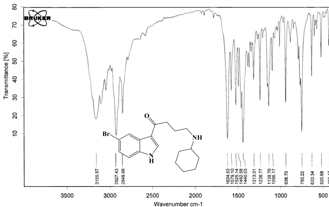
FT-IR SPECTRUM
