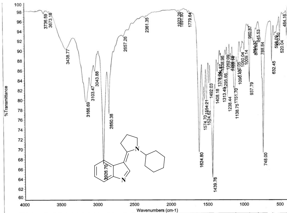
FT-IR SPECTRUM
