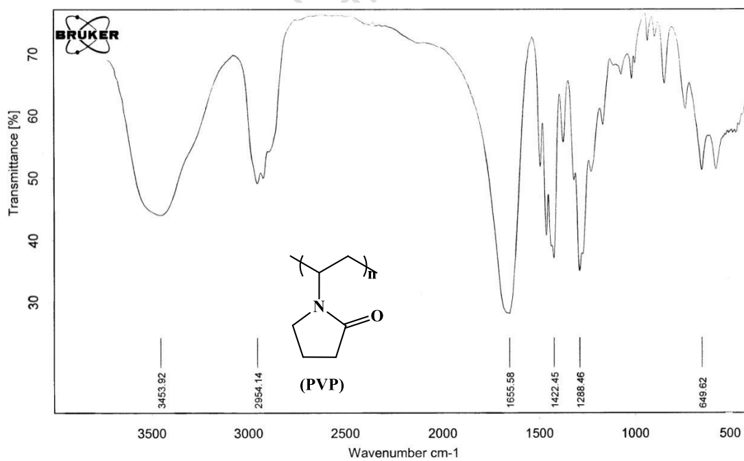
FT-IR SPECTRUM
