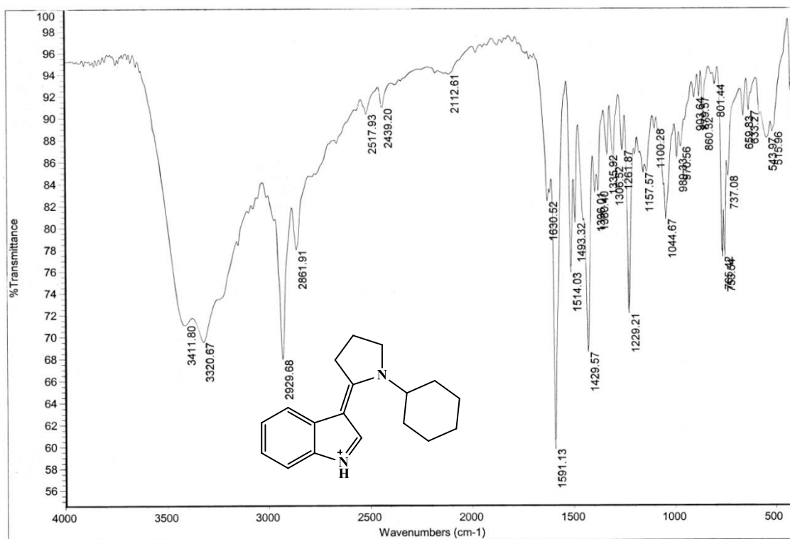
FT-IR SPECTRUM
