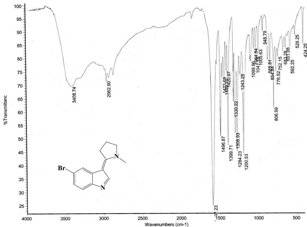
FT-IR SPECTRUM
