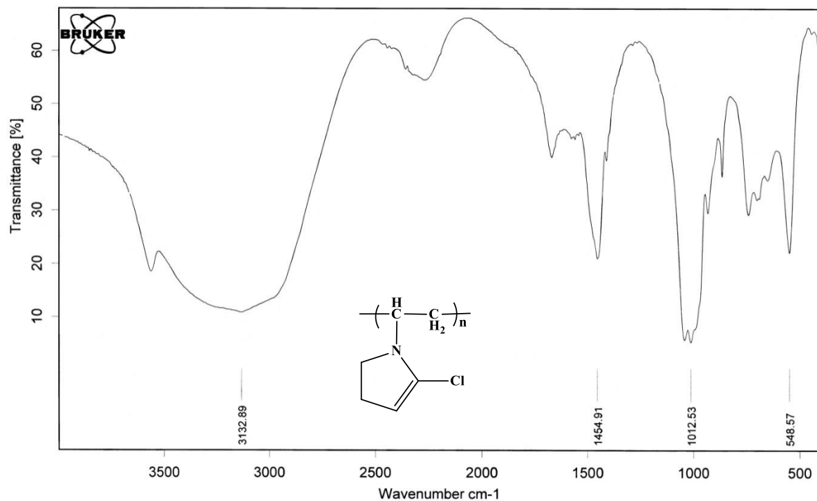
FT-IR SPECTRUM
