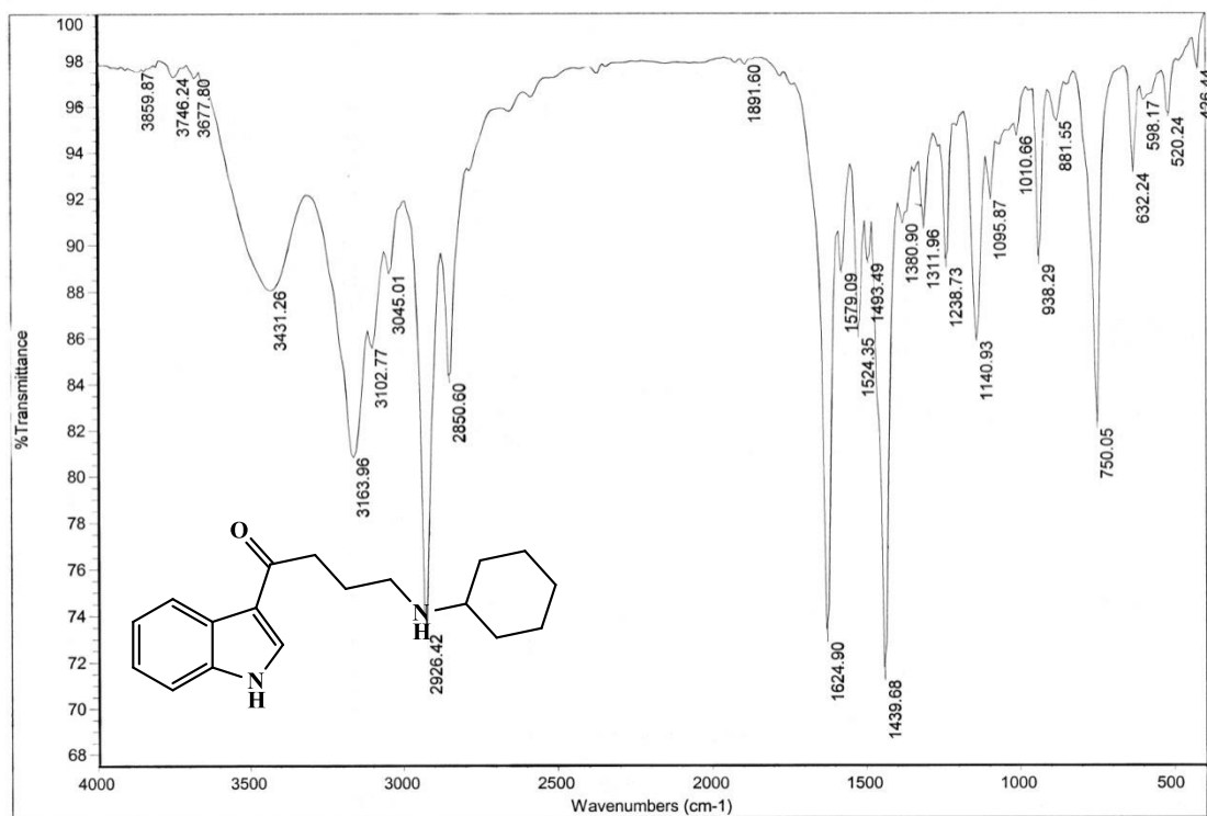
FT-IR SPECTRUM
