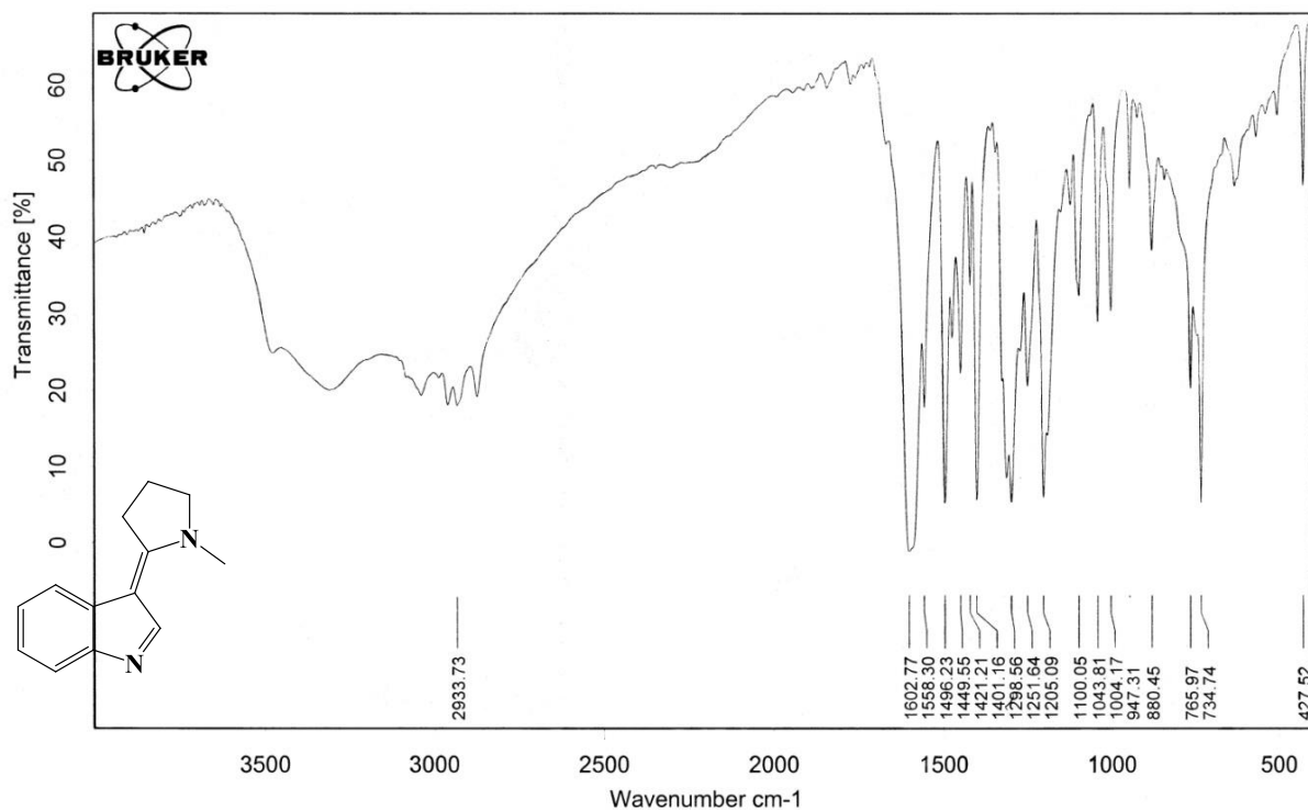
FT-IR SPECTRUM
