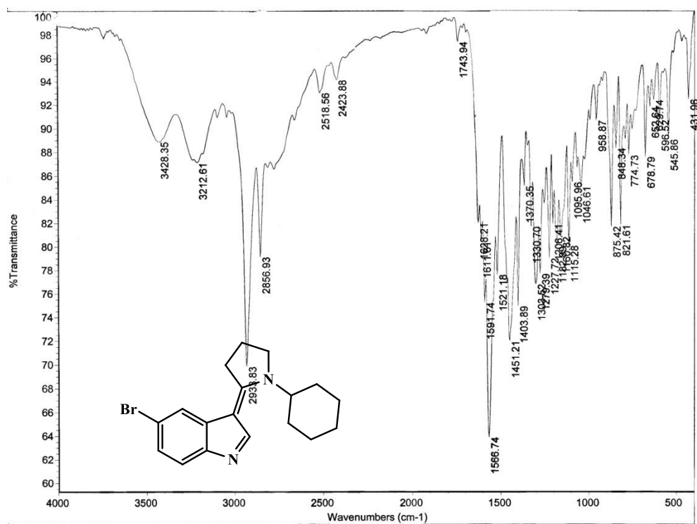
FT-IR SPECTRUM
