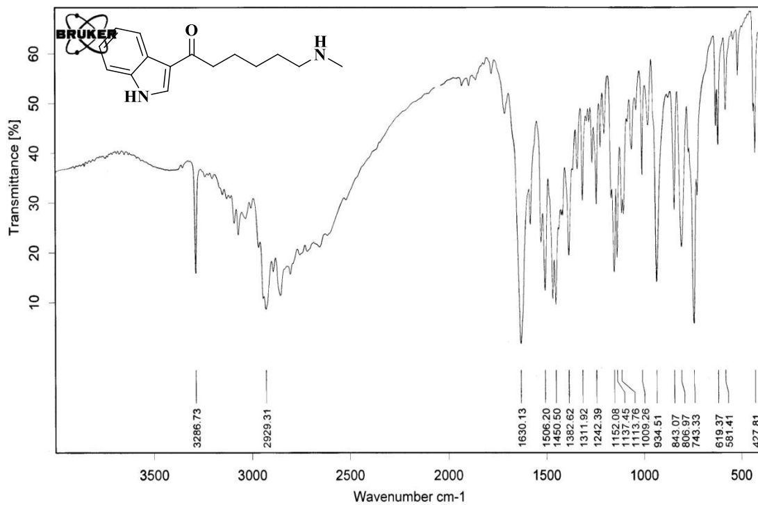
FT-IR SPECTRUM
