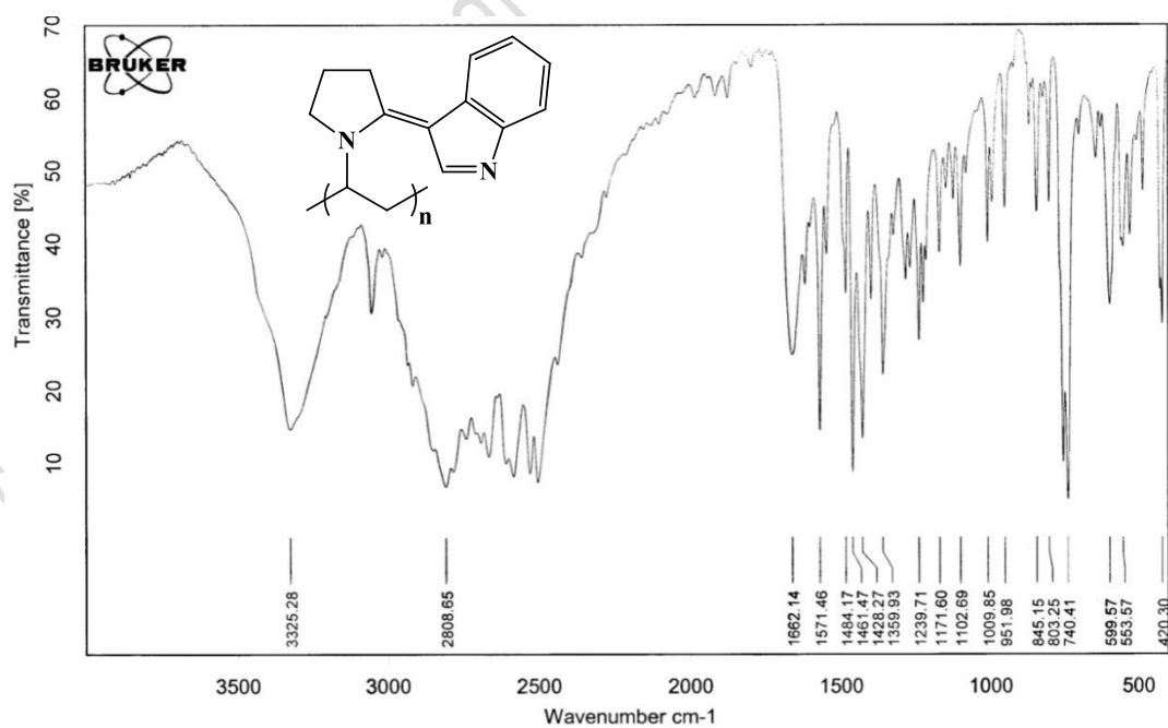
FT-IR SPECTRUM
